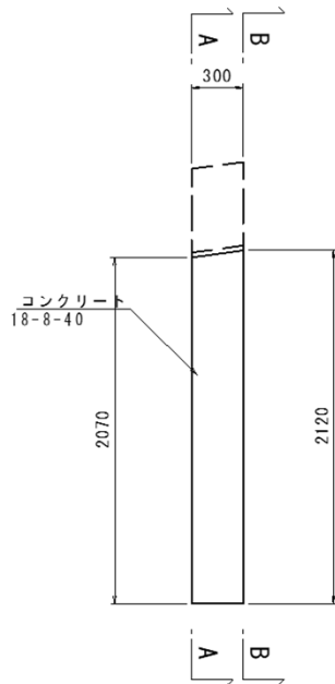
正面図
